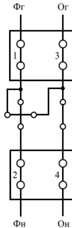
Рис. Г.2. Схема подключения счетчика «АТЛАС1» без размыкателя или с внешним УЗО
