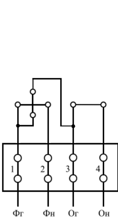
Рис. Г.1. Схема подключения счетчика «АТЛАС1» с размыкателем
