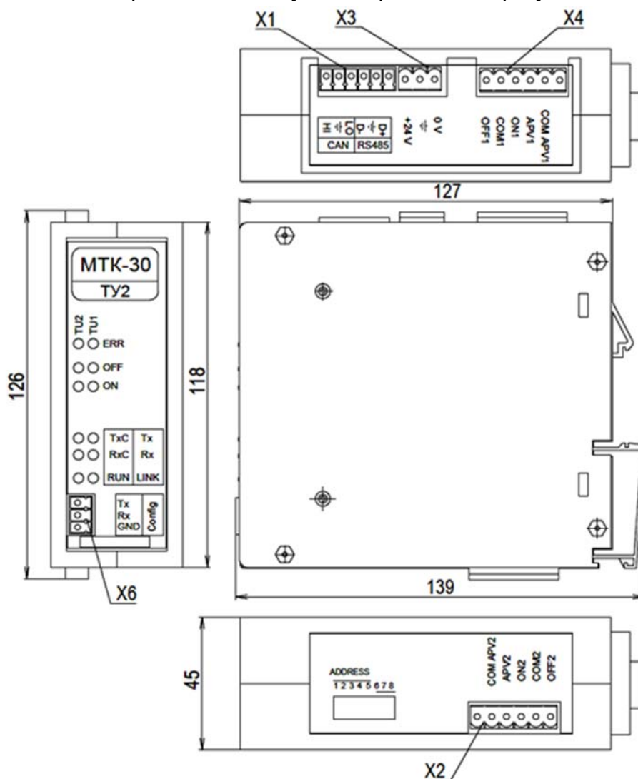
Рисунок 1 – Расположение разъемов на модуле ТУ
